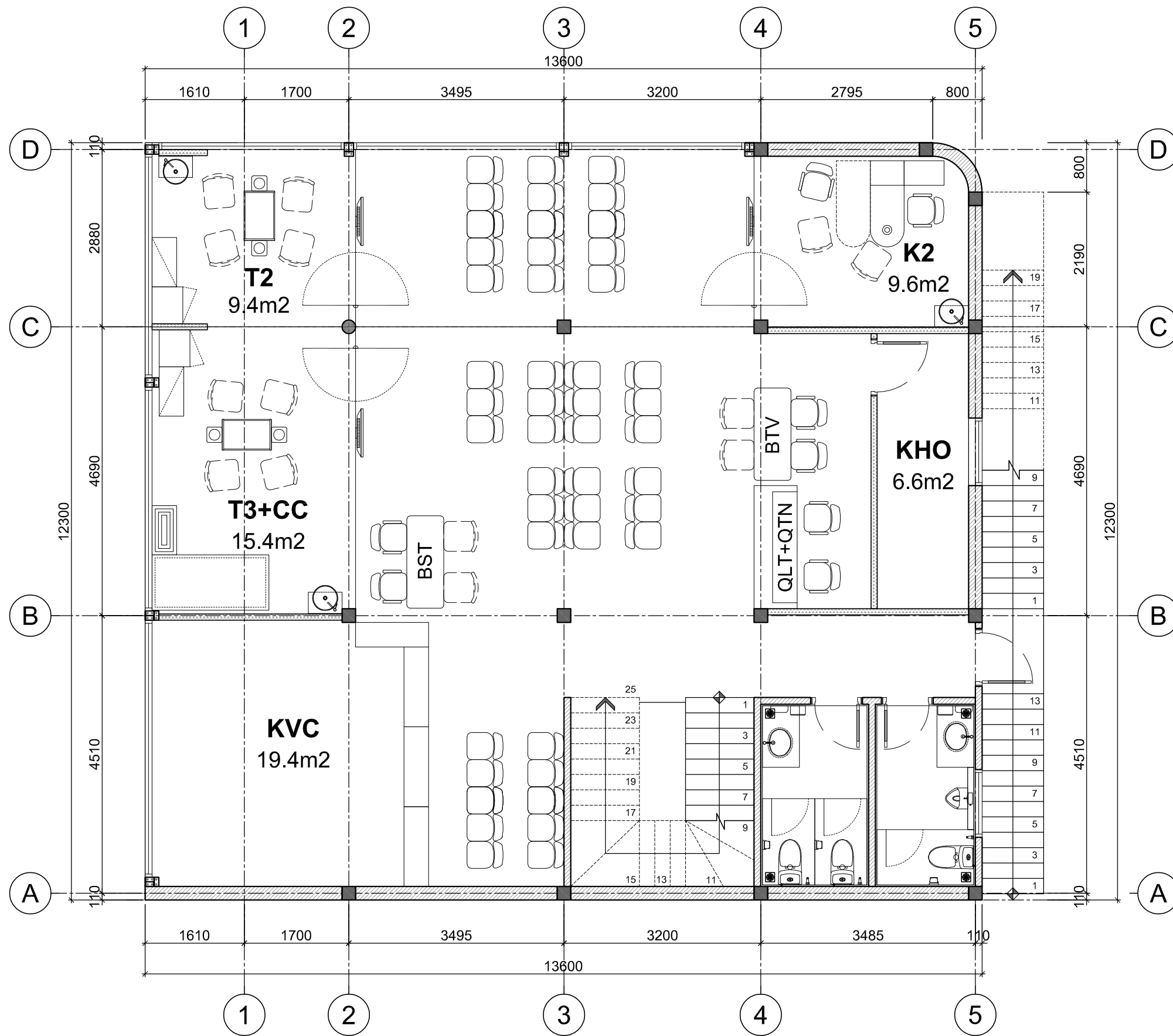
LAYOUT MẶT BẰNG TẦNG 2
